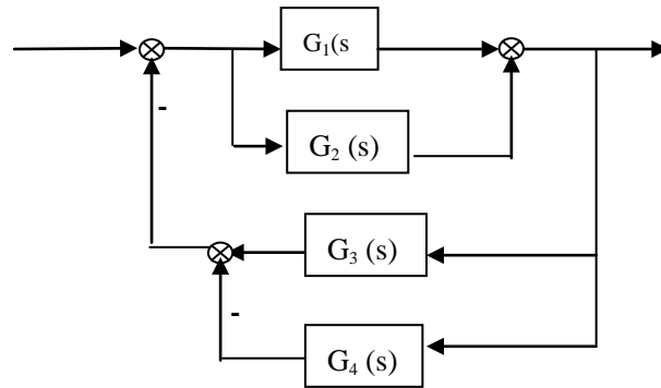
图 6.4 结构框图
