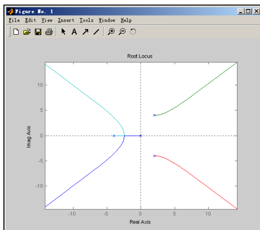
图 6.18 根轨迹
