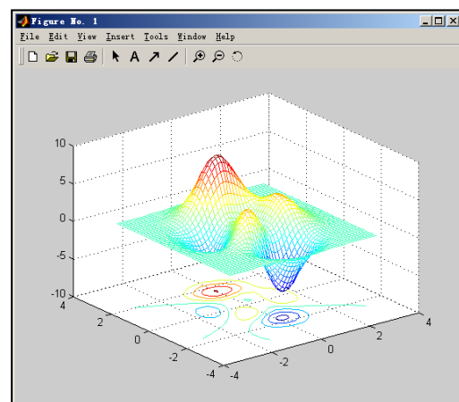
图 4.17 (b) peaks 函数的曲面图加等高线
