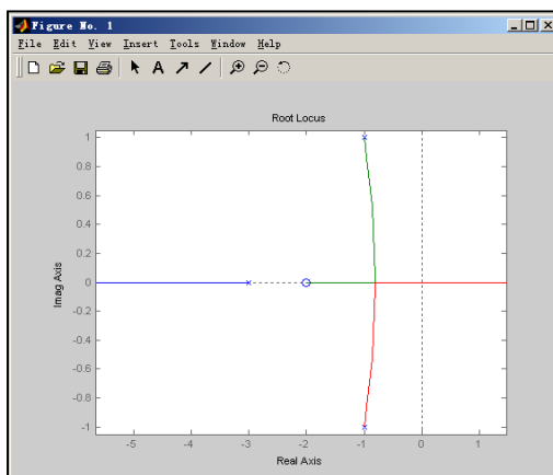
图 6.19 零度根轨迹
