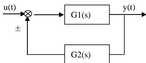
图 6.3 反馈结构
