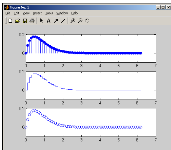
图 4.27 离散数据图
