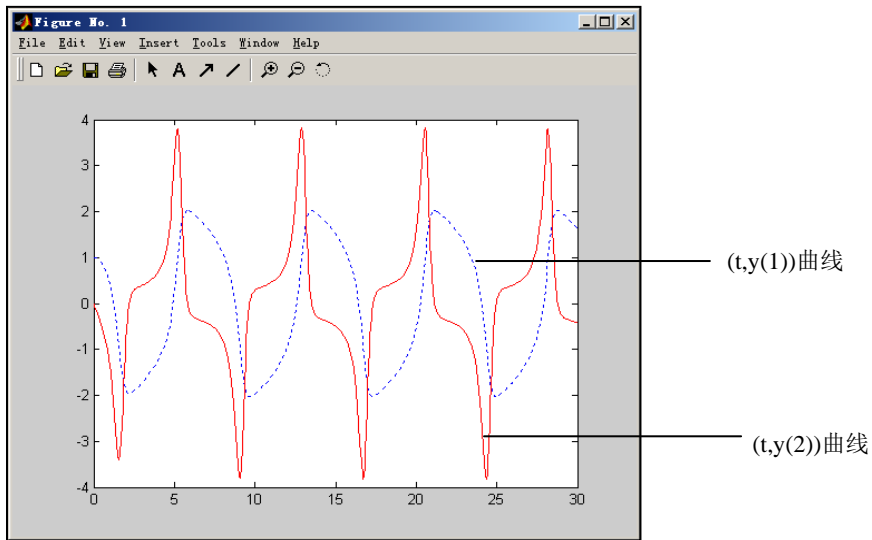
图 5.9 微分方程解
