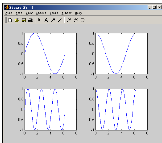
图 4.6 四个子图
