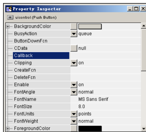
图 4.50 属性编辑器
