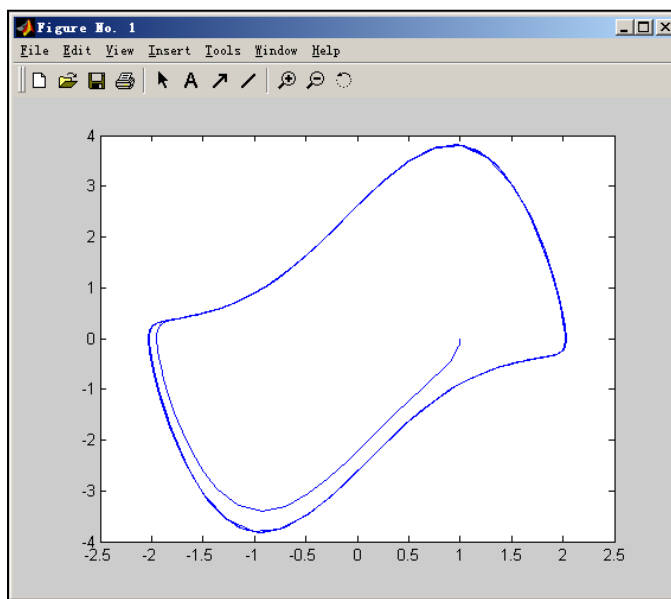
图 5.10 相平面图
