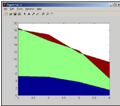
图 4.24 (a) 面积图
