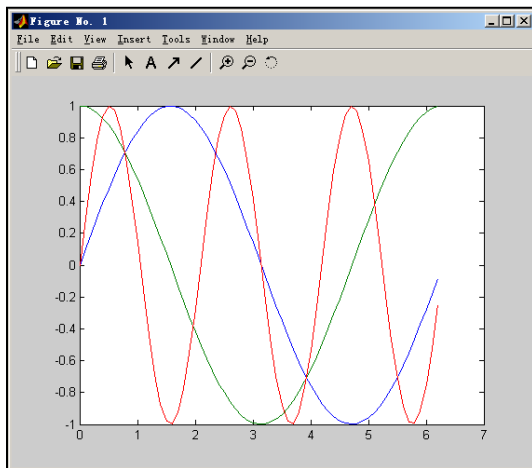
图 4.5 三条曲线
