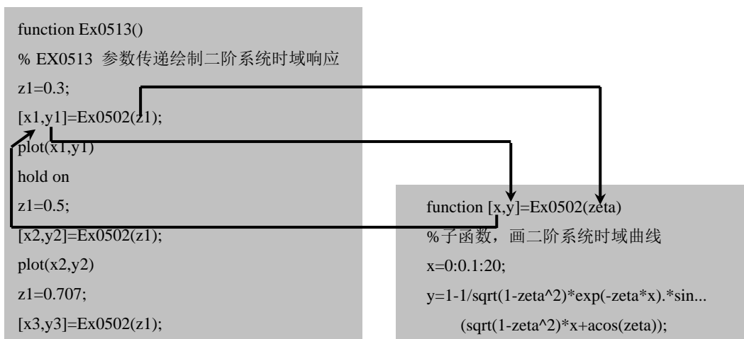
图 5.3 参数传递
