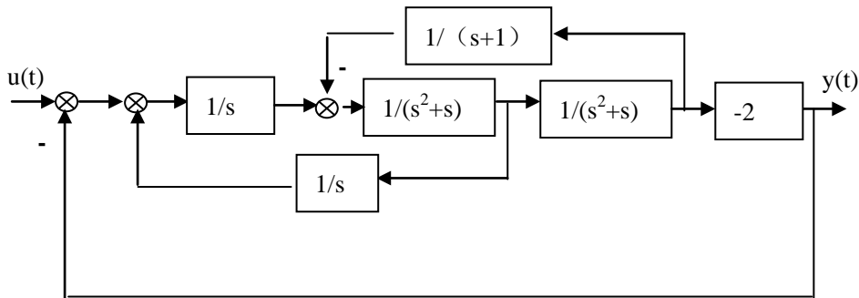
图 6.5 结构框图
