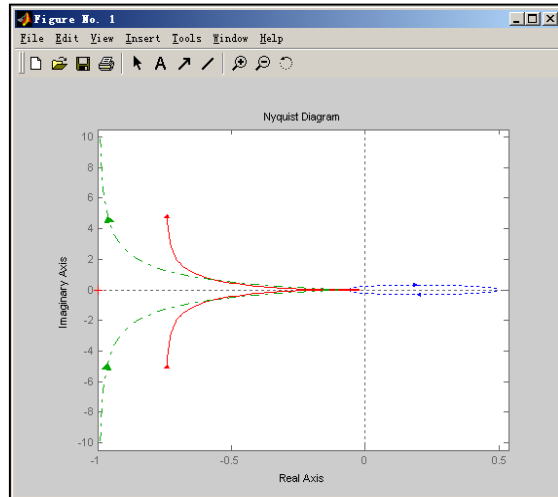
图 6.15 nyquist 曲线
