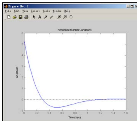
图 6.7 零输入响应曲线
