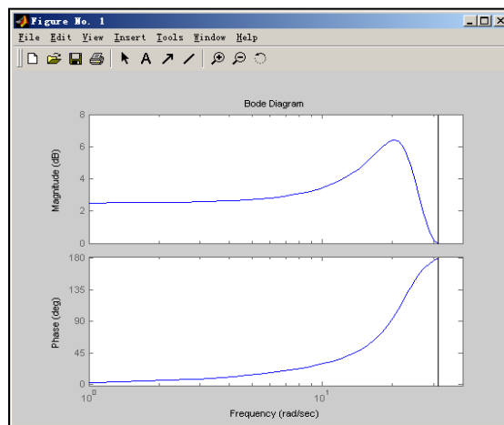
图 6.17 离散系统的 bode 图
