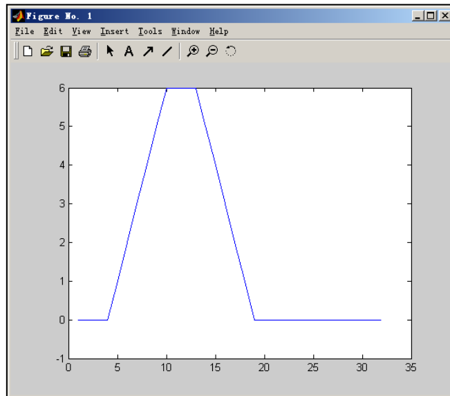
图 2.10 卷积结果
