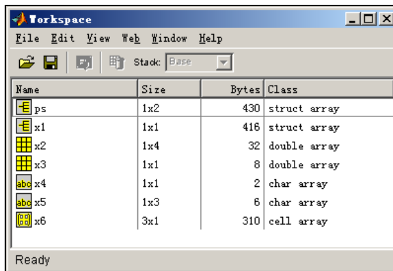
图 2.8 工作空间
