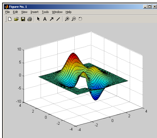
图 4.20 peaks 函数
