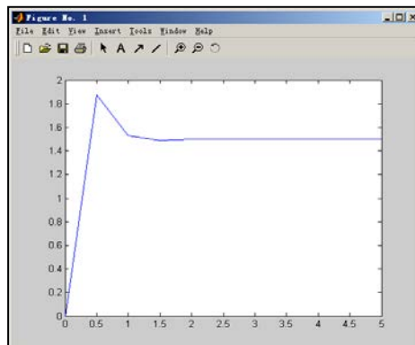
图 6.11 (b) 步长增大的阶跃响应曲线
